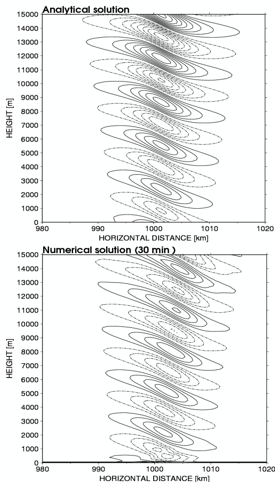
図1. 山岳波の上方伝播に関する数値実験．等値線は w を表す．実線が正、破線が負の値．0.05m/s 毎．上図が解析解，下図が本研究で開発したモデルの数値解．
